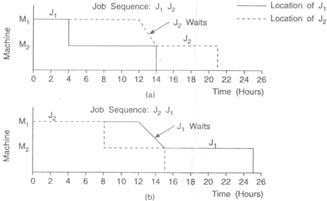
Fig. 2.8.9 Gantt Chart
